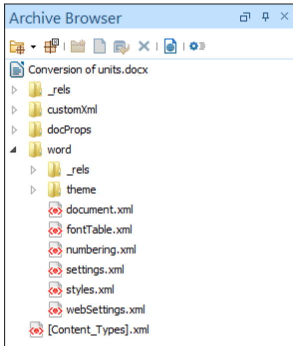
Figure 324. Archive Browser
